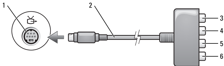
1 S 视频电视输出连接器 2 分量视频适配器 3 S/PDIF 数字音频连接器 4 Pr (红色) 分量视频输出连接器 5 Pb (蓝色) 分量视频输出连接器 6 Y (绿色) 分量视频输出连接器
