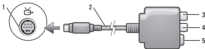
1 S 视频电视输出连接器 2 复合视频适配器 3 S/PDIF 数字音频连接器 4 复合视频输出连接器 5 S 视频连接器
